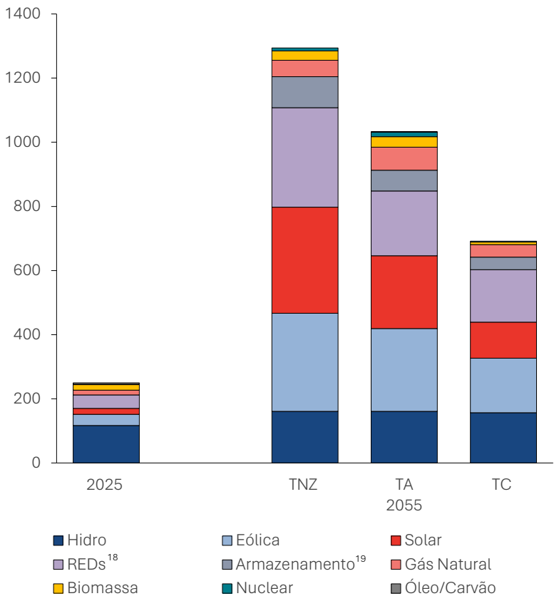
Capacidade instalada total do sistema elétrico em 2055 (GW) 17
