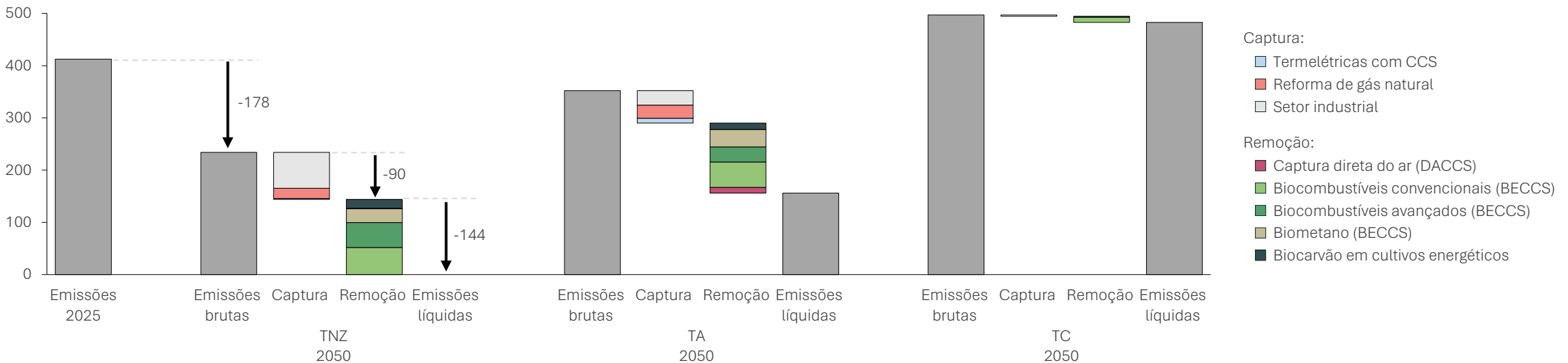
Emissões líquidas de GEE do setor de energia (milhões de toneladas de CO 2 equivalente)
