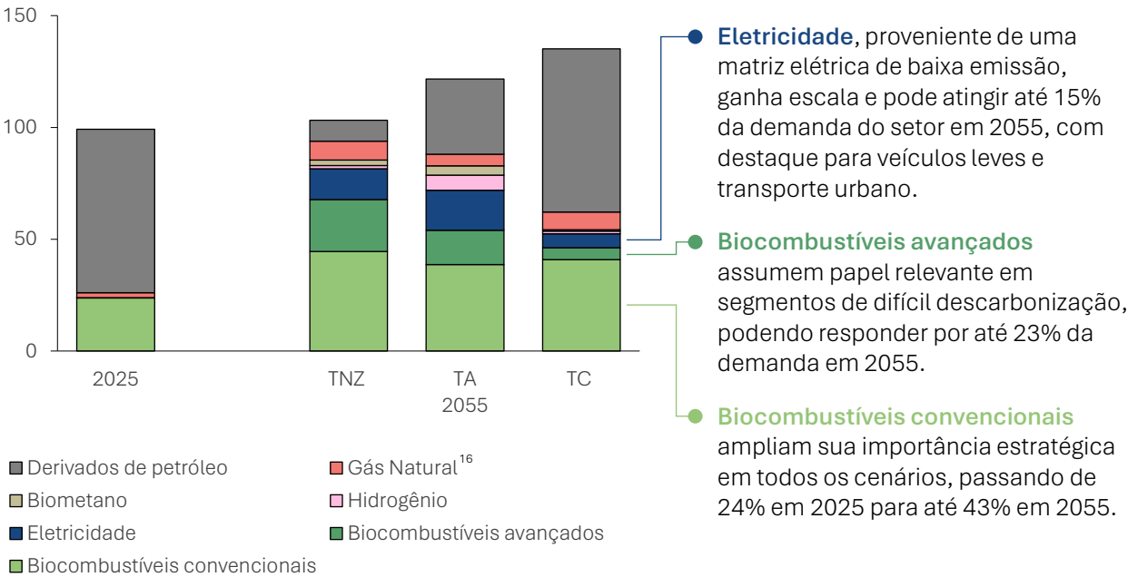
Demanda de energia do setor de transportes por fonte (milhões de tep)
