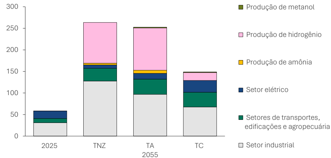
Demanda de gás natural e biometano (milhões m³/d)
