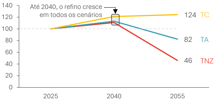
Produção das refinarias brasileiras (2025 = base 100)
