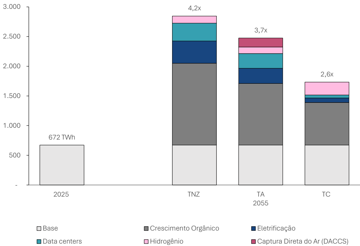
Composição da carga de energia elétrica em 2055 (TWh)
