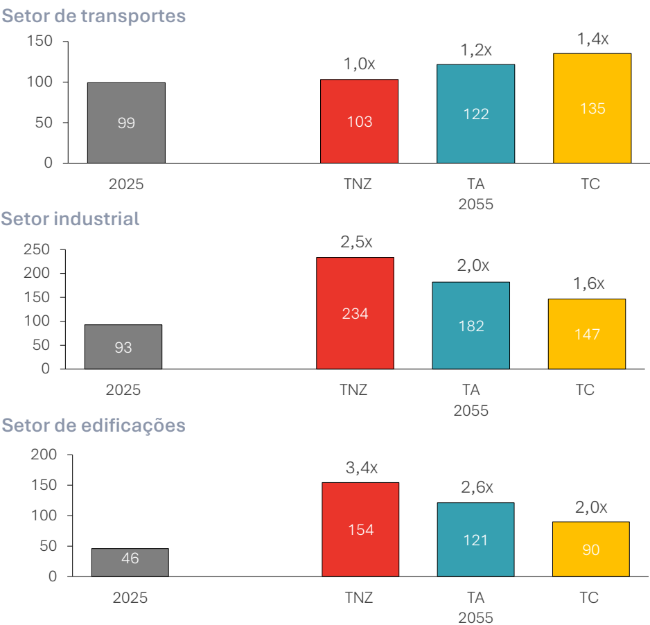
Demanda de energia de setores selecionados (milhões de tep)
