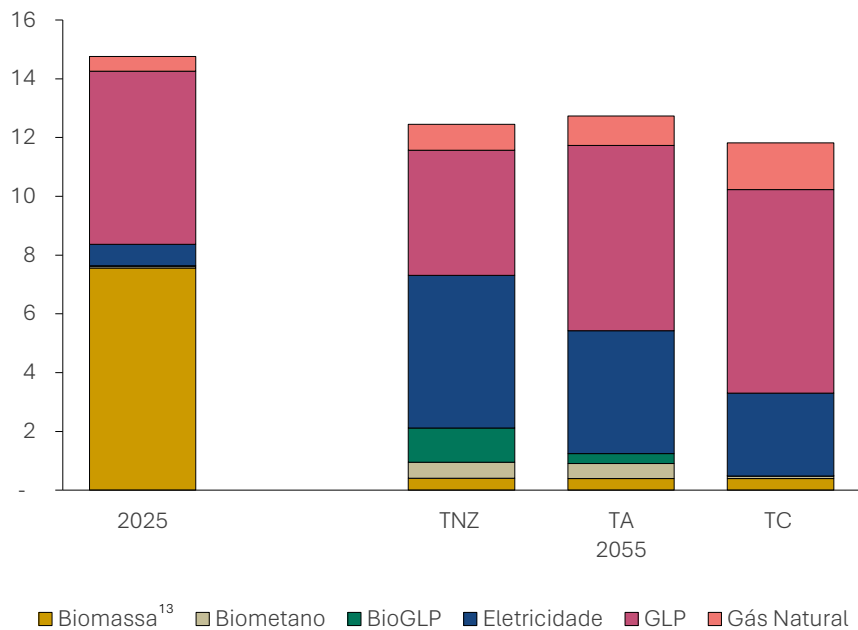
Consumo energético no cozimento de alimentos (milhões tep)
