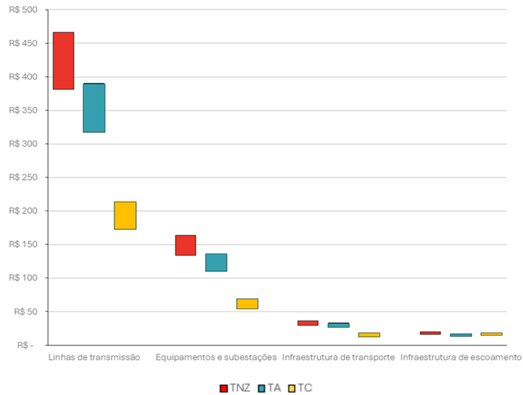
Investimentos em infraestruturas do setor energético 36 (R$ bilhões)
