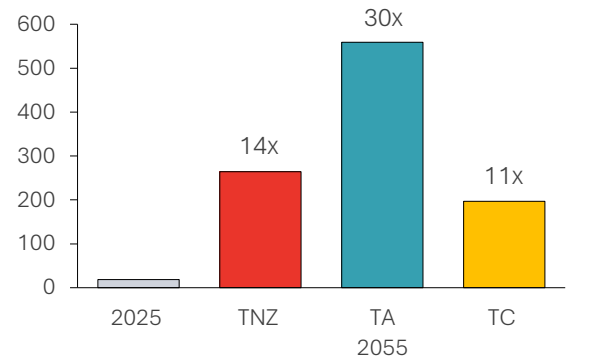
Minerais estratégicos em baterias para eletromobilidade (mil toneladas)
