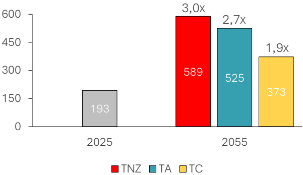
Evolução da extensão de linhas de transmissão (mil km)
