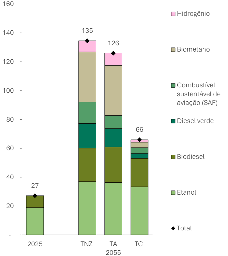
Produção de biocombustíveis (milhões de tep)
