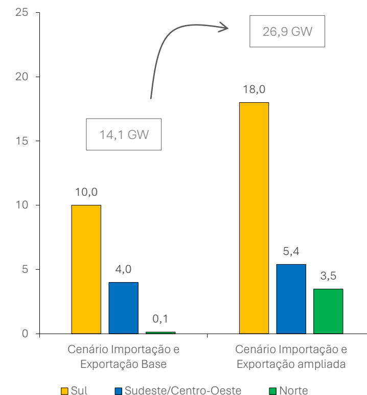
Estimativa da capacidade das interligações internacionais em 2055 (GW)
