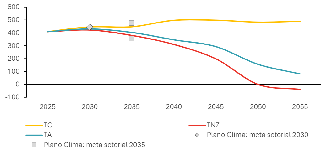
Emissões líquidas e metas de emissões de GEE 30 do setor de energia (milhões de toneladas de CO 2 equivalente)
