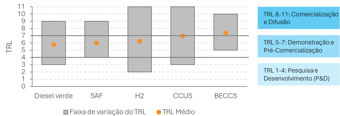
Nível de maturidade de tecnologias emergentes selecionadas
