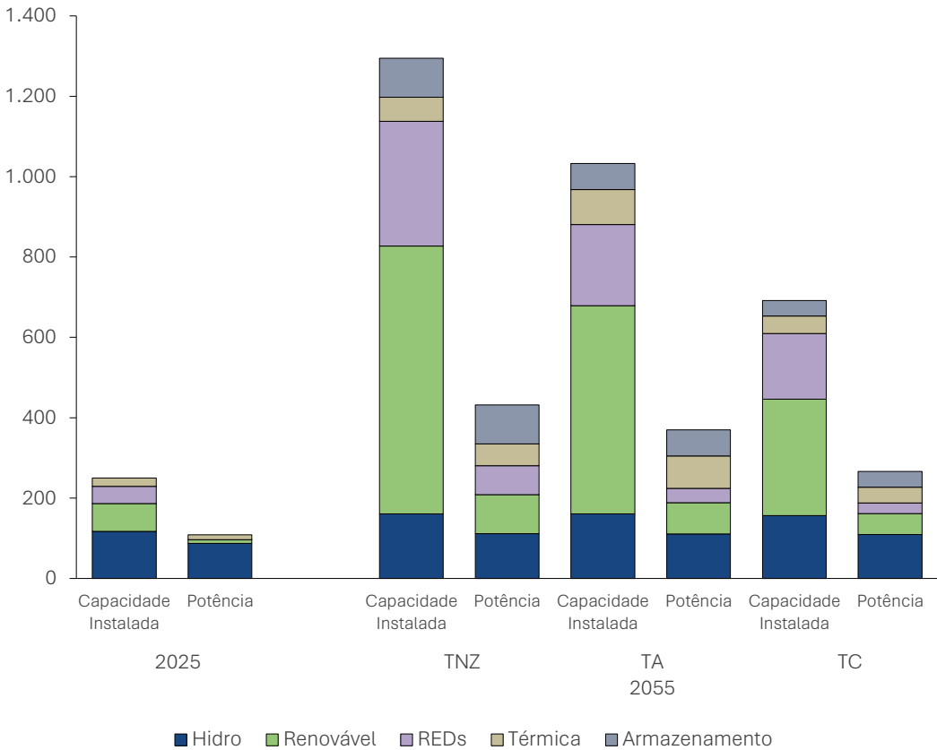
Participação das fontes na capacidade instalada e disponibilidade de potência 26 (GW)
